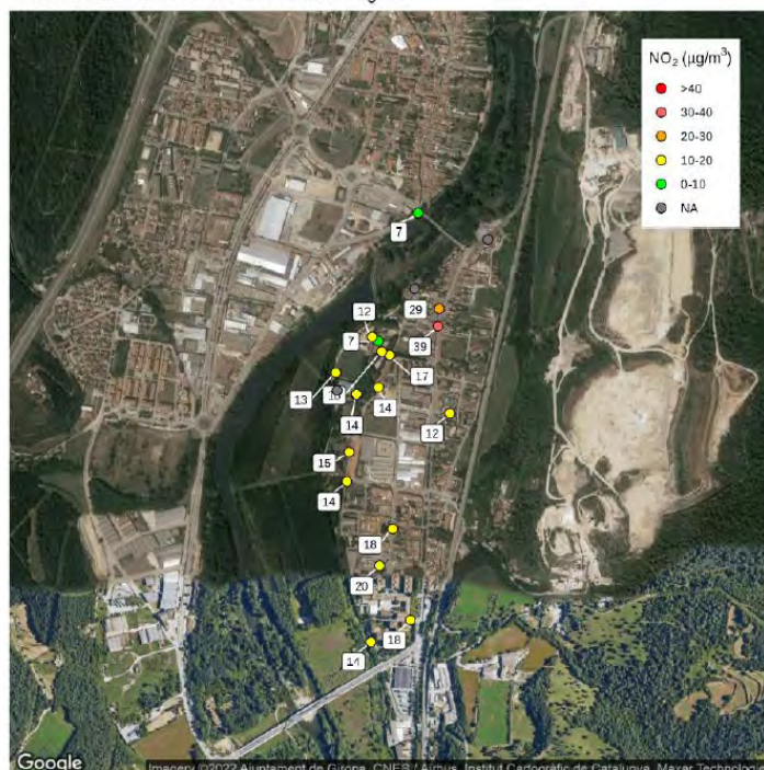
Concentracions de NO 2 a l'Escola Carme August
