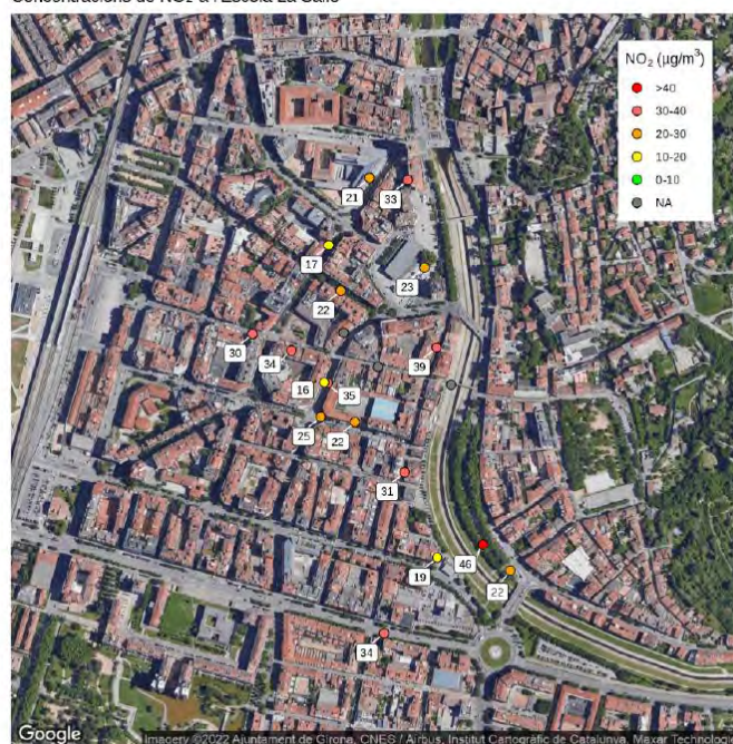
Concentracions de NO 2 a l'Escola La Salle
