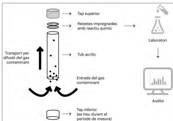
Dosímetre passiu de NO 2 del tipus Palmes (Font: 4SFERA)
