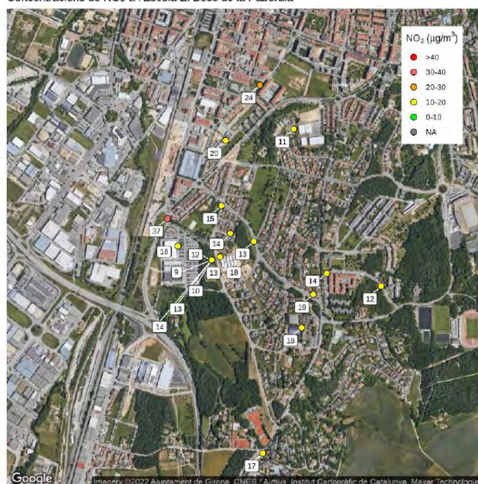
Concentracions de NO 2 a l'Escola El Bosc de la Pabordia
