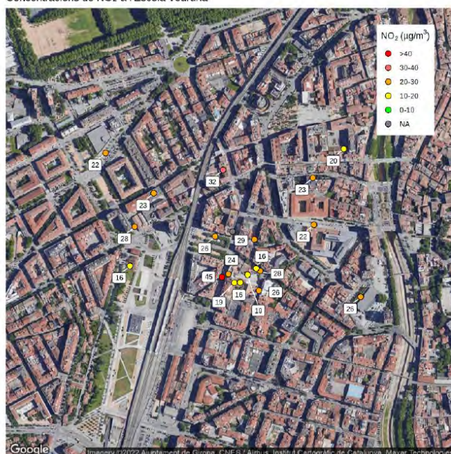
Concentracions de NO 2 a l'Escola Vedruna
