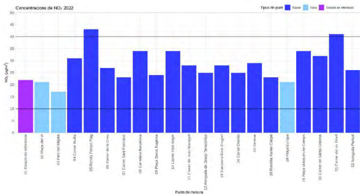
Concentracions de NO 2 obtingudes (Font: 4SFERA)
