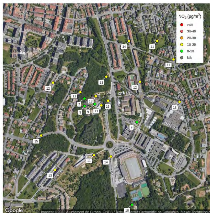
Concentracions de NO 2 a l'Escola Font de l'Abella
