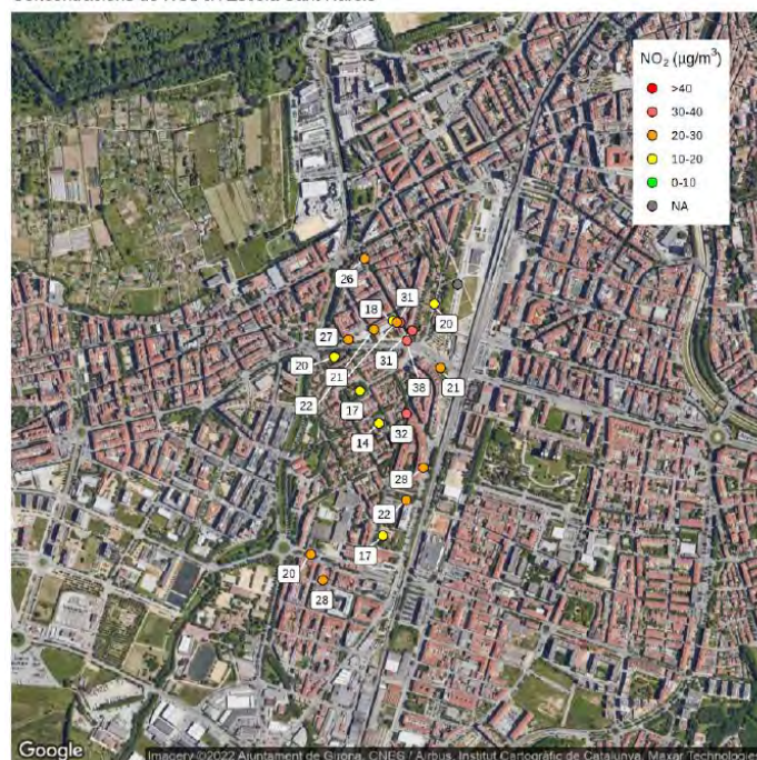
Concentracions de NO 2 a l'Escola Sant Narcís
