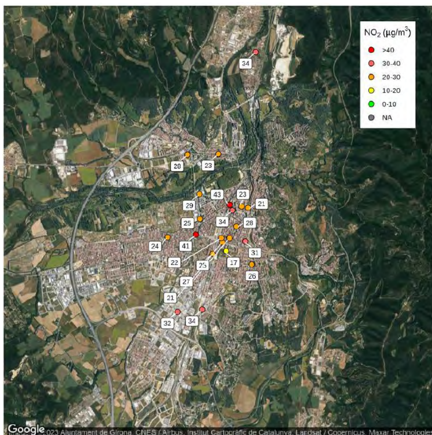
Concentracions de NO 2 obtingudes (Font: 4SFERA)
