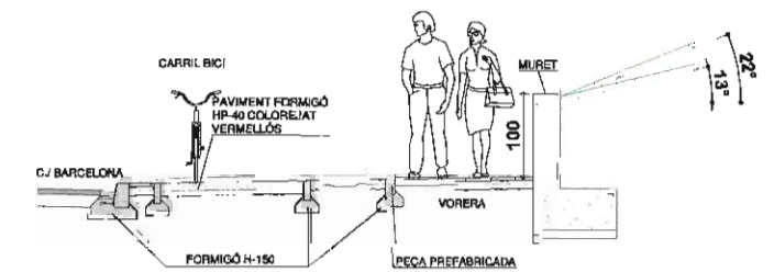
SECCIÓ PROLONGACIÓ VORERA C./ BARCELONA ESC.: 1/100
