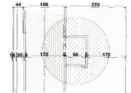
PLANTA PROLONGACIÓ VORERA C./ BARCELONA ESC.: 1/100
