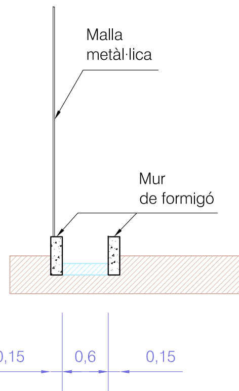
A2.2 SECCIÓ 1-1 Escala 1/50
