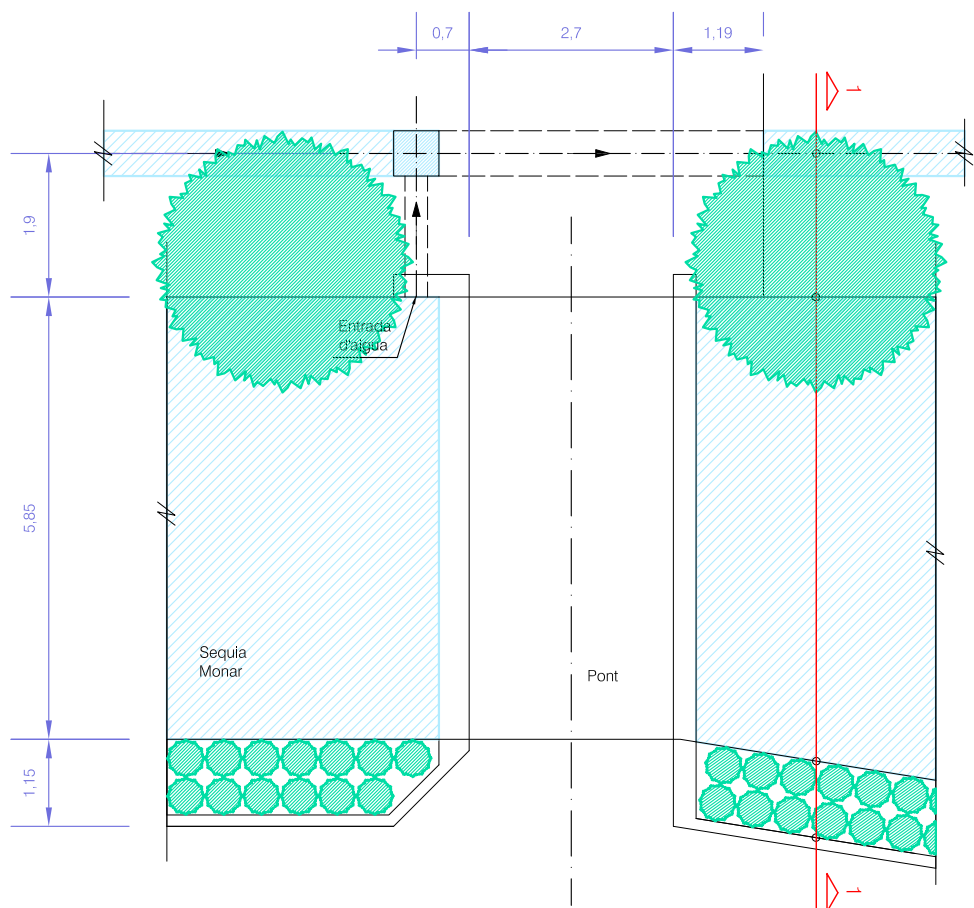
A1.1 PLANTA Escala 1/100
