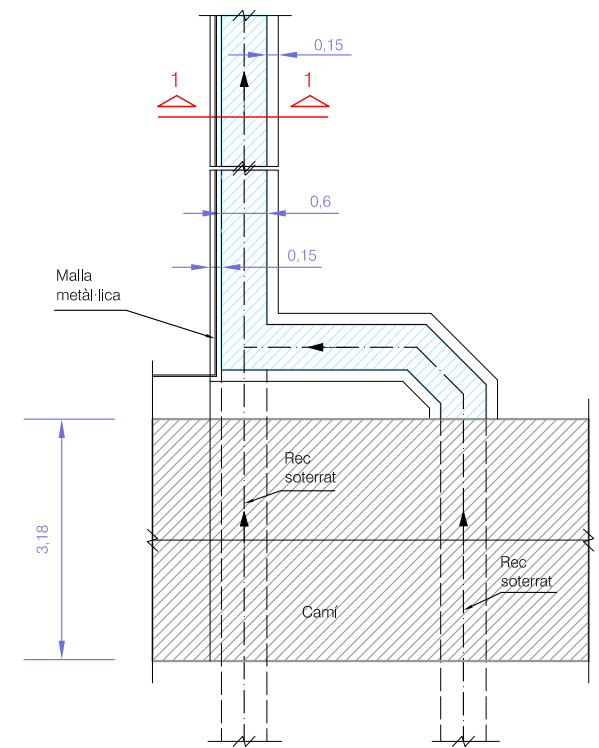
A2.1 PLANTA Escala 1/100
