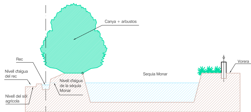
A1.2 SECCIÓ 1-1 Escala 1/100
