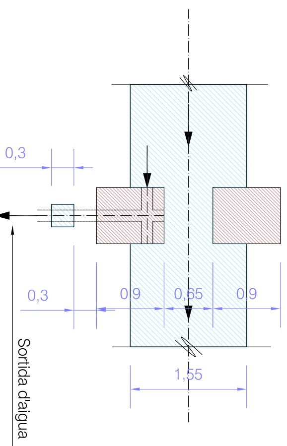
C4.4 PLANTA Escala 1/50
