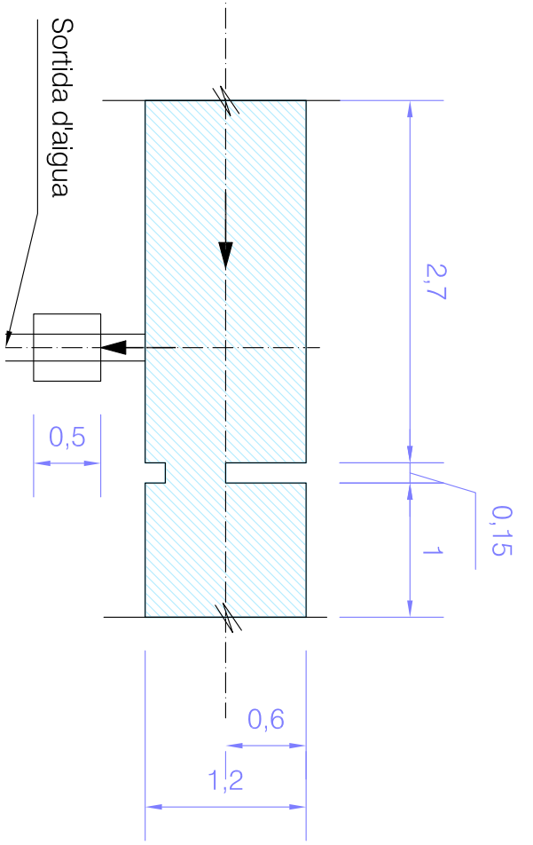
C4.1.1 PLANTA 1-1 Escala 1/50
