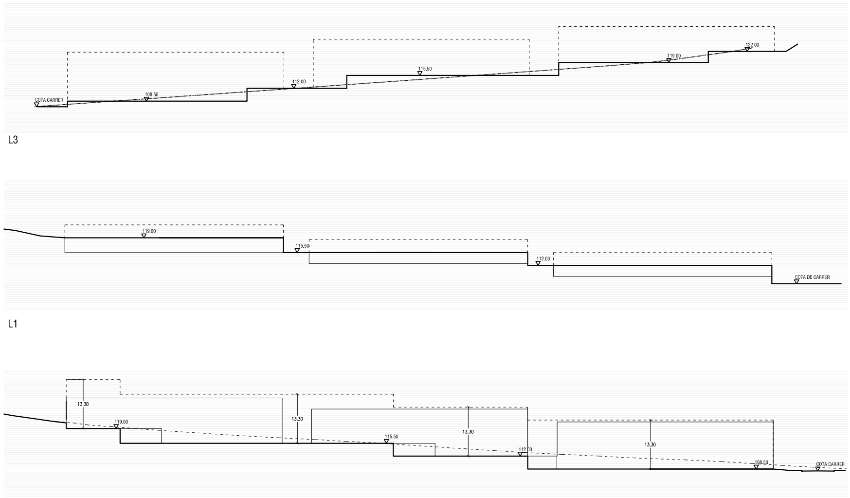
SECCIONS LONGITUDINAL - DEFINICIÓ DE RASANTS E 1:1000
