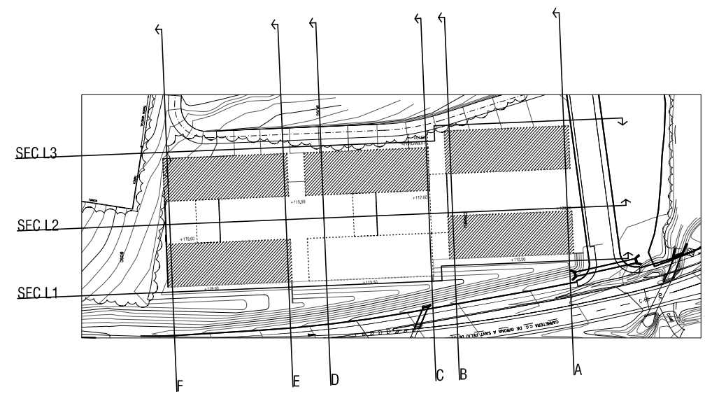
SECCIONS LONGITUDINAL - DEFINICIÓ DE RASANTS E 1:1000
