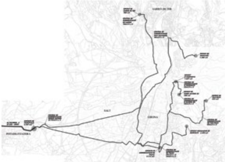
Esquema actual de la xarxa bàsica d'abastament d'aigua potable des del Pasteral a l'àrea metropolitana de Girona. Font: Aigües de Girona, Salt i Sarrià
