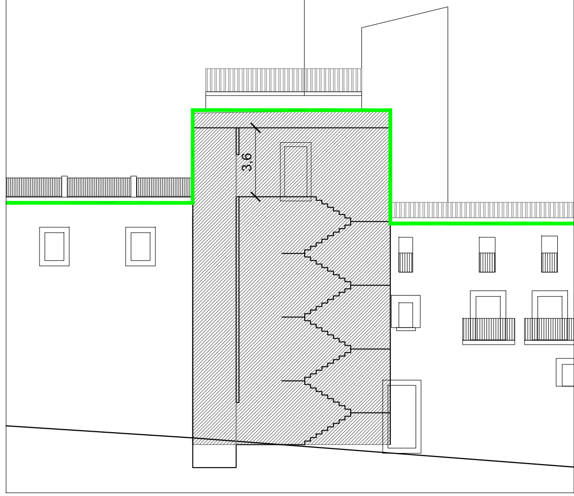
SECCIÓ NUCLI ACCESSOS
