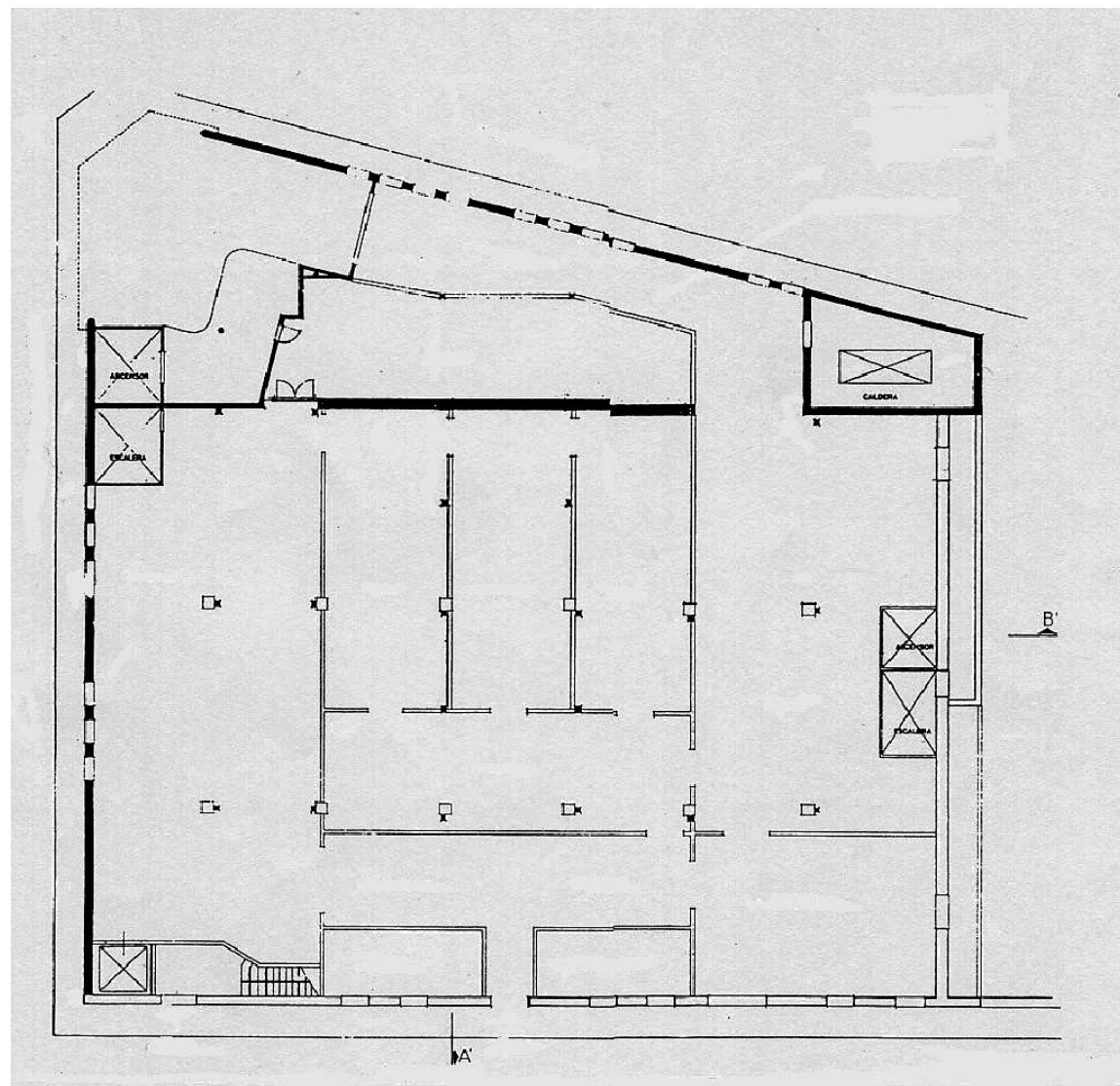
PLANTA BAIXA
