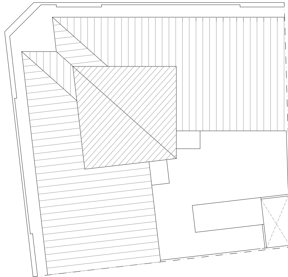
Planta Coberta
