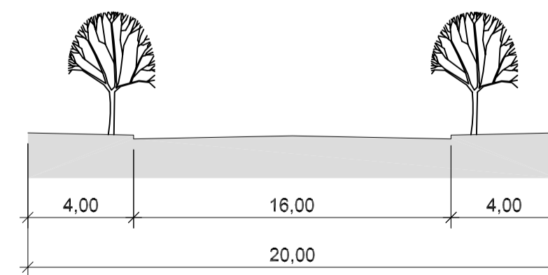
SECCIÓ A-A
