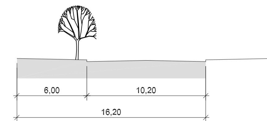
SECCIÓ B-B
